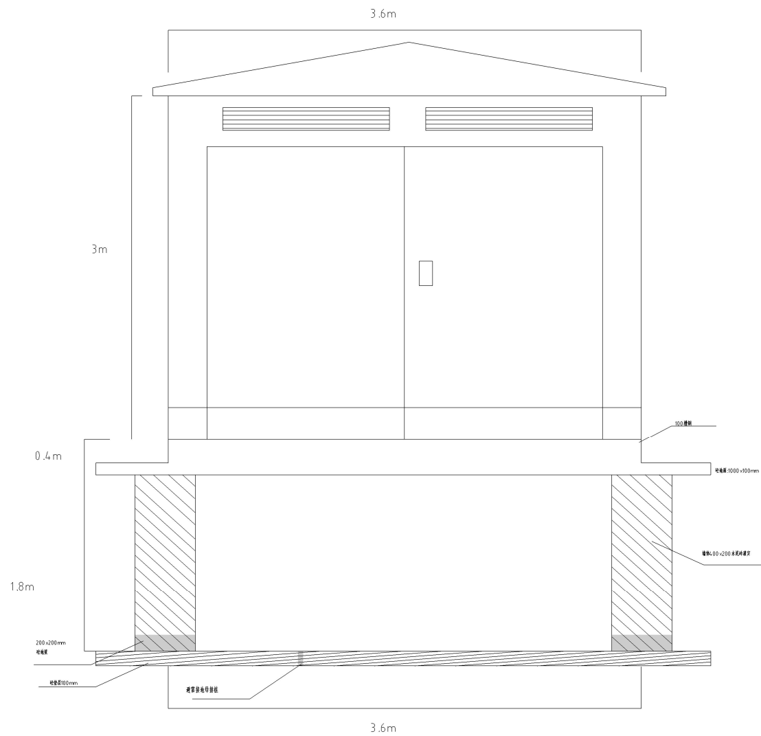
箱变基础示意图
